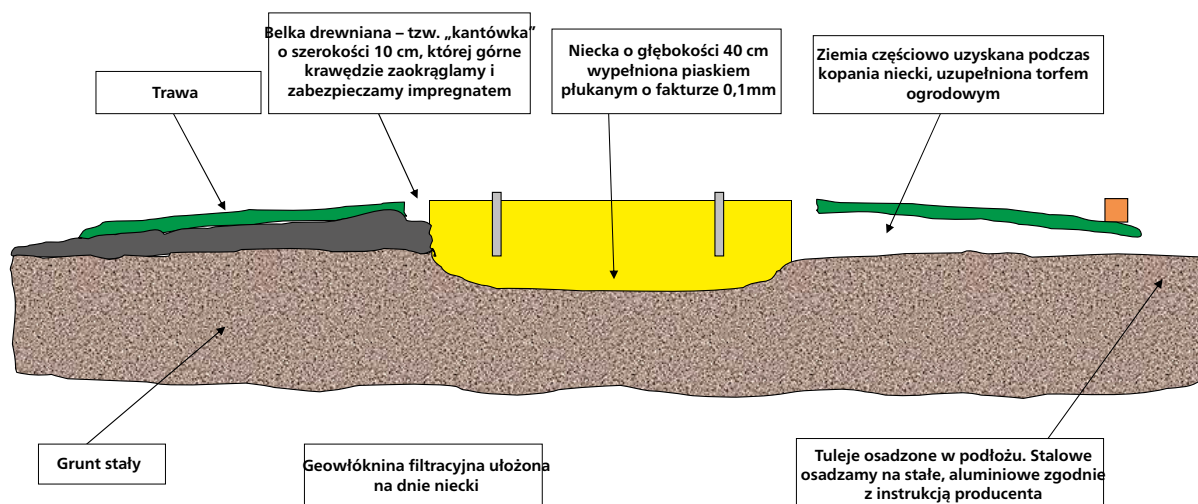
RYСУNEK 5. BUDOWA BOISKA
